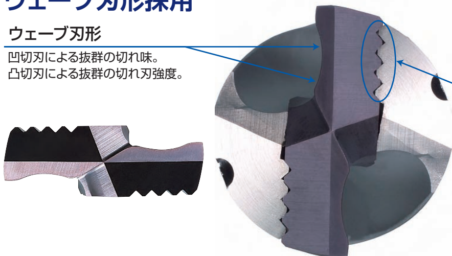
切刃形状
